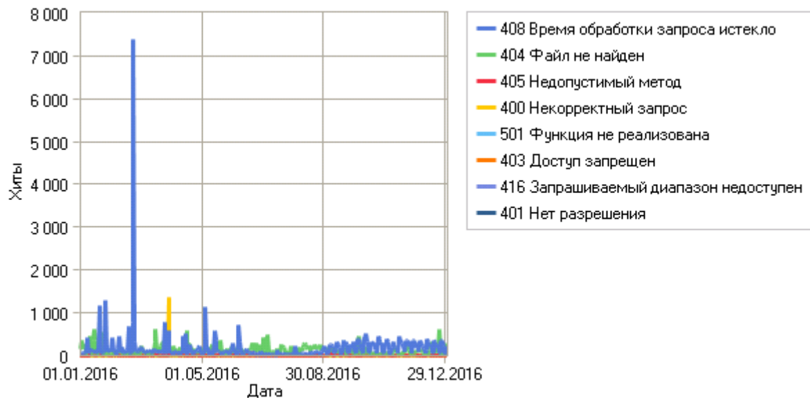
Типы ошибок
