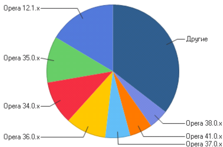
Версии Опера
