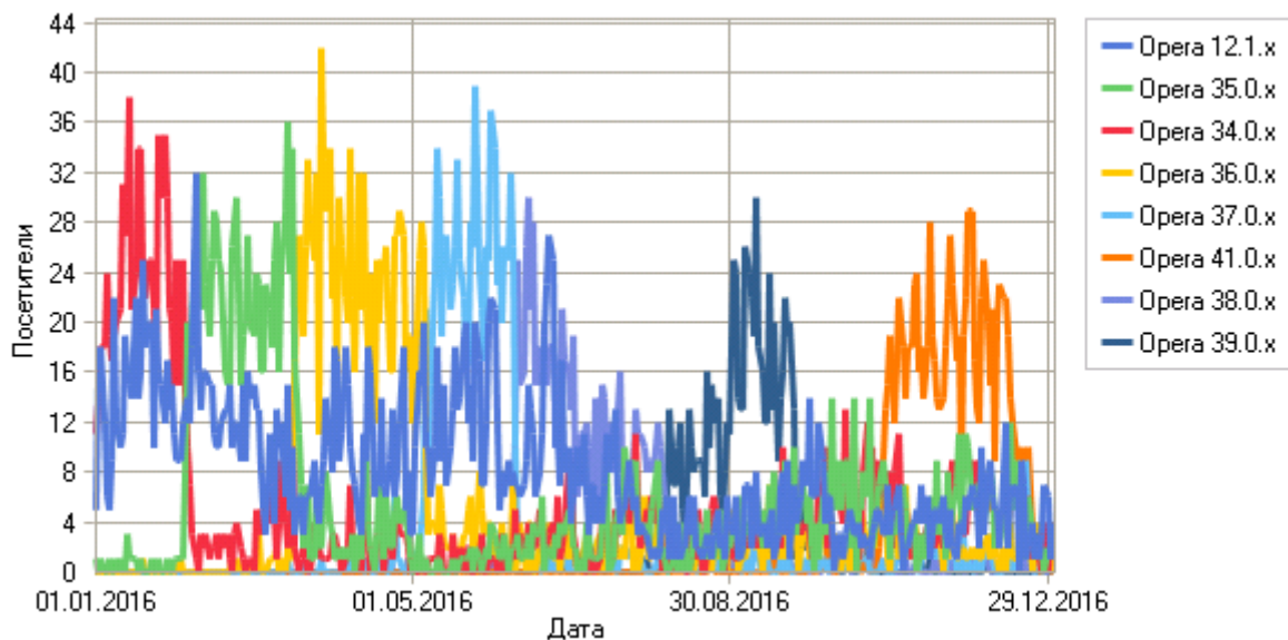
Версии Опера
